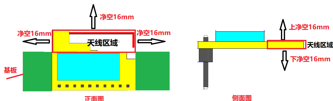
Figure 9. 模组建议放置区域
