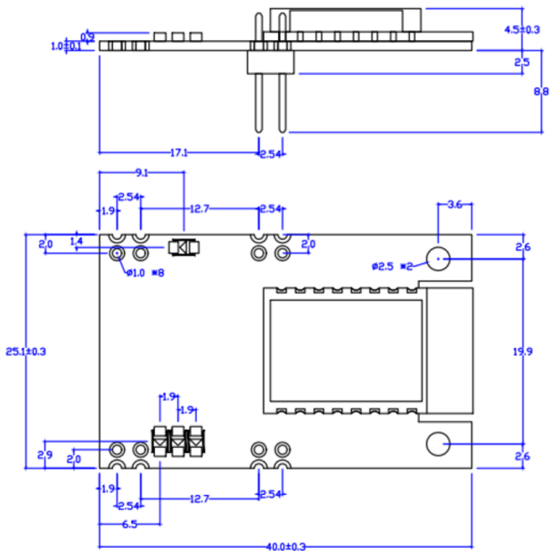
Figure 7. Wport-W71-AA-1/0(2M)机械尺寸
