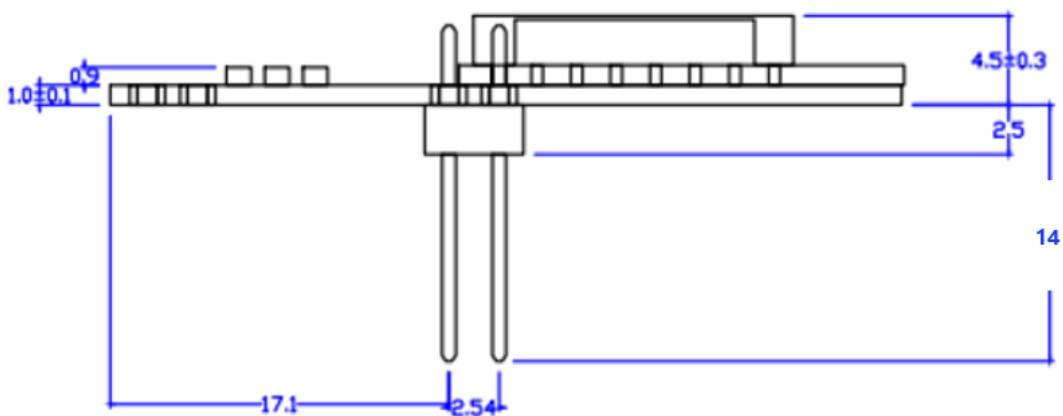
Figure 8. Wport-W71-AA-1/0(2ML)机械尺寸
