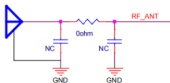
Figure 6. 外置天线焊盘推荐电路
