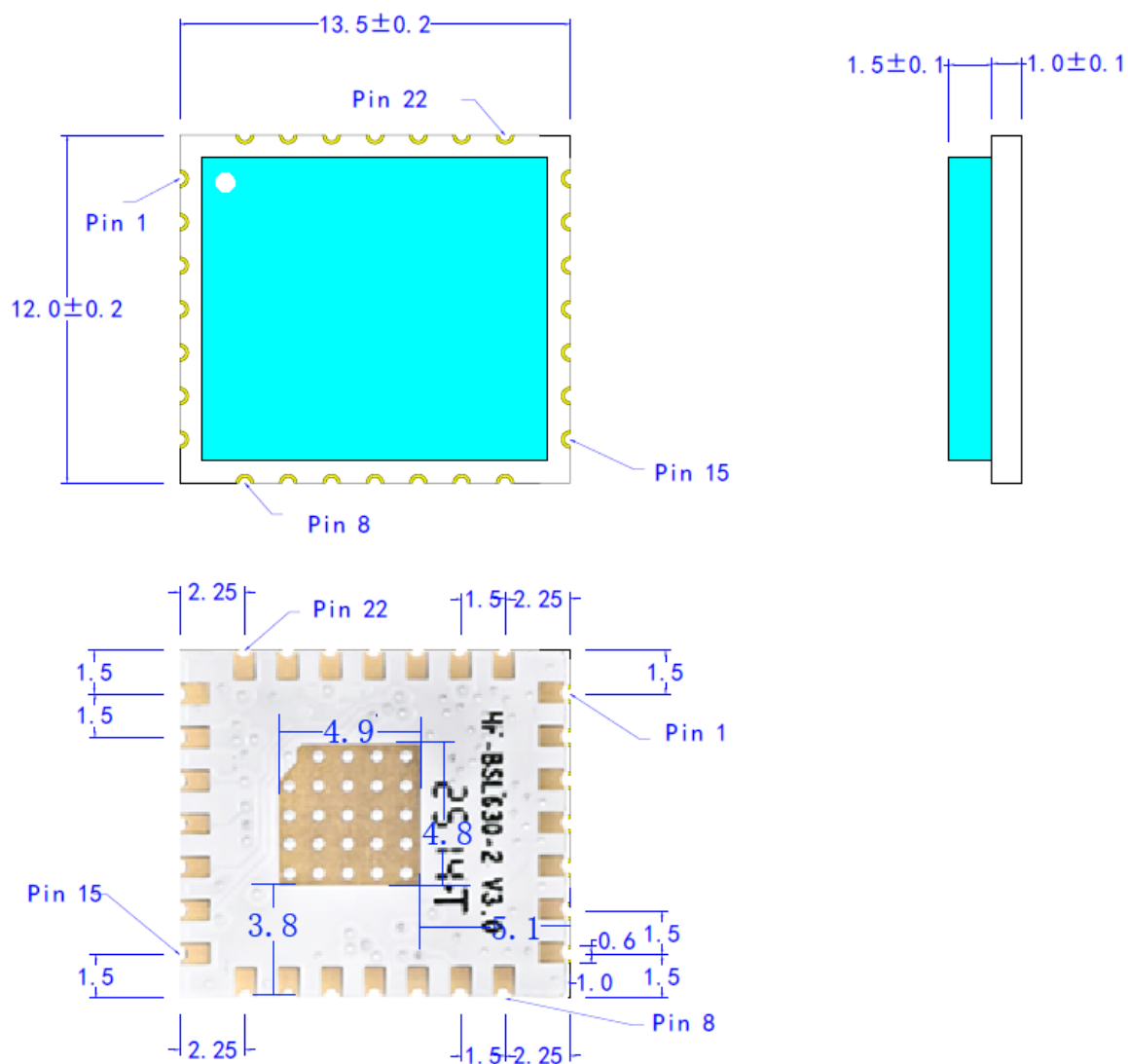
Figure 4. 机械尺寸
