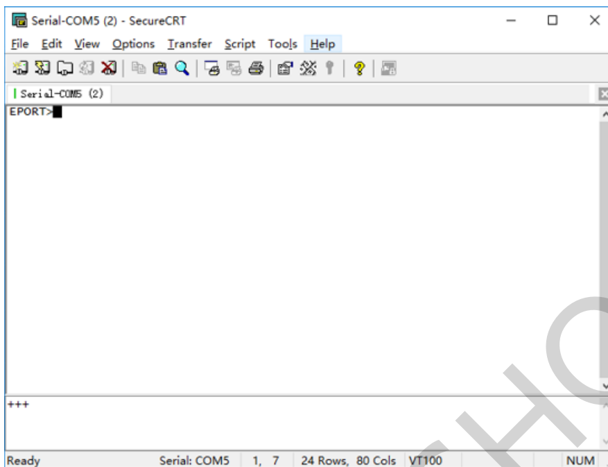
Figure 48. 从透传模式切换到命令模式
