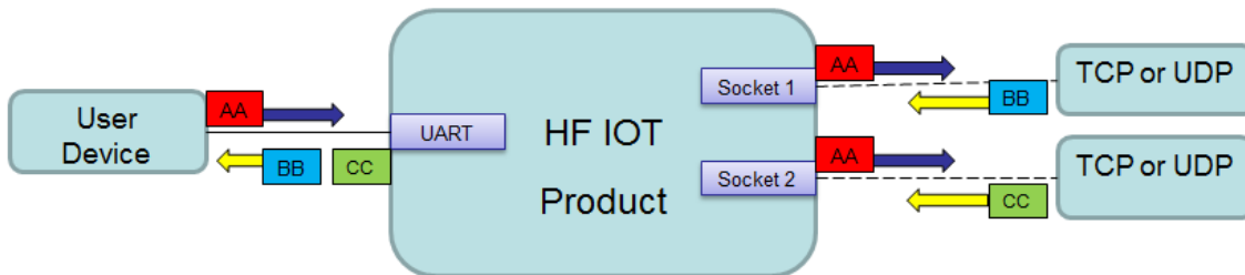
Figure 15. 多 Socket 数据传输样例
