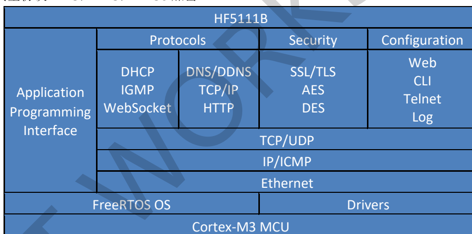
Figure 10. HF5111B 系列 软件协议架构图
