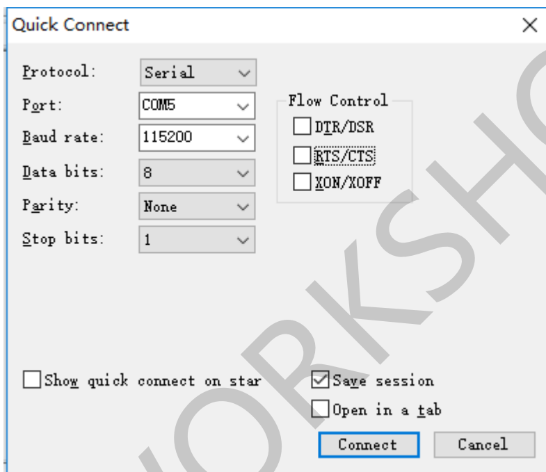
Figure 47. HFXXXX 系列缺省 UART 参数
