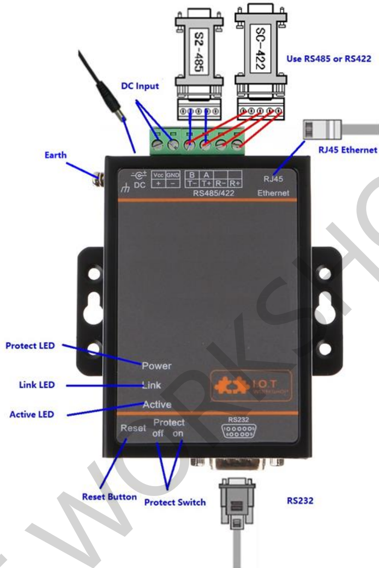
Figure 2. HF5111B 正面图
