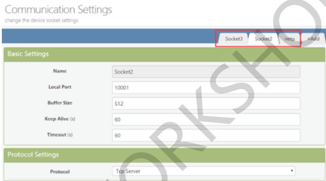
Figure 16. 网页创建多 Socket 通道
