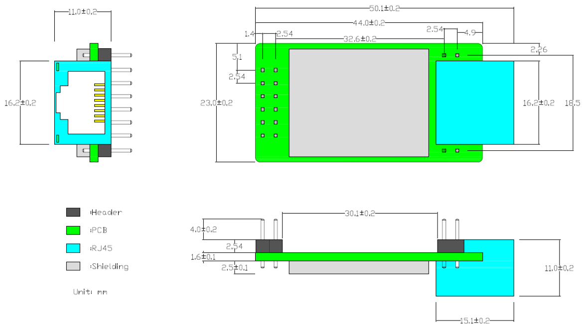
Figure 5. Eport Pro-EP20 系列机械尺寸
