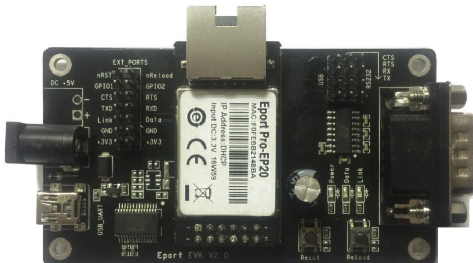
Figure 8. Eport Pro-EP20 系列 EVK 评估套件
