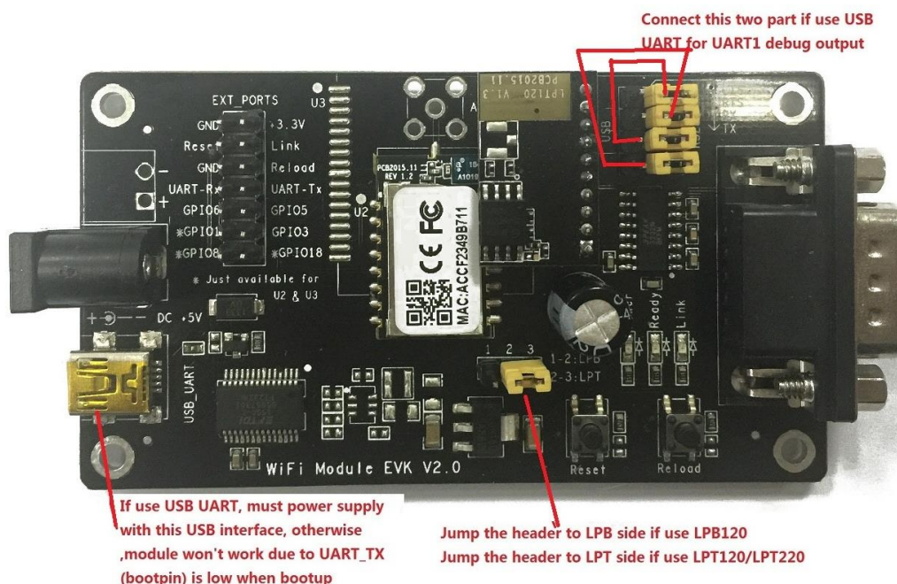
Figure 6. LPT120/LPT220 开发板
