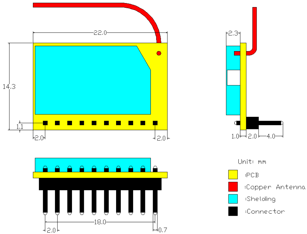
Figure 3. HF-LPT120A 机械尺寸
