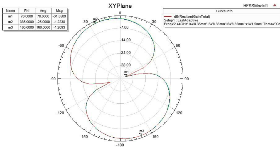
Figure 12. HF-LPT120XY 平面辐射方向图
