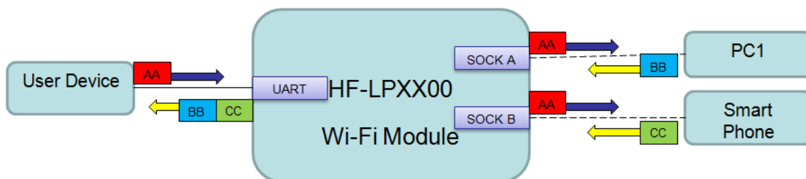
Figure 18. 双 Socket 数据流向示意图
