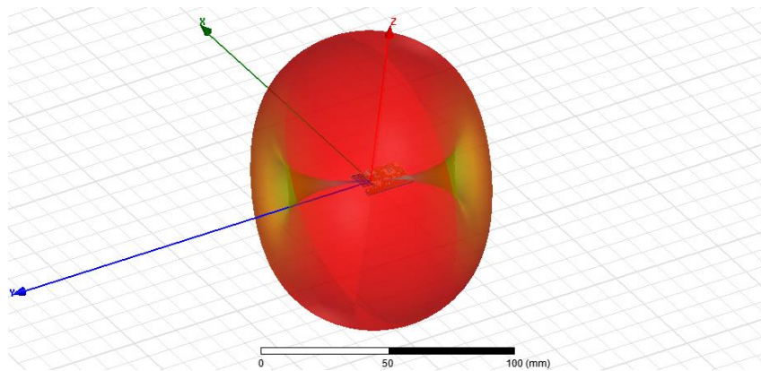
Figure 11. HF-LPT120 天线辐射方向图
