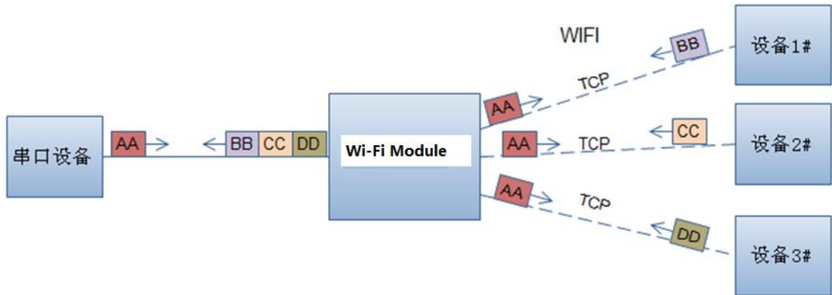
Figure 19. 多 TCP 链接数据传输图示
