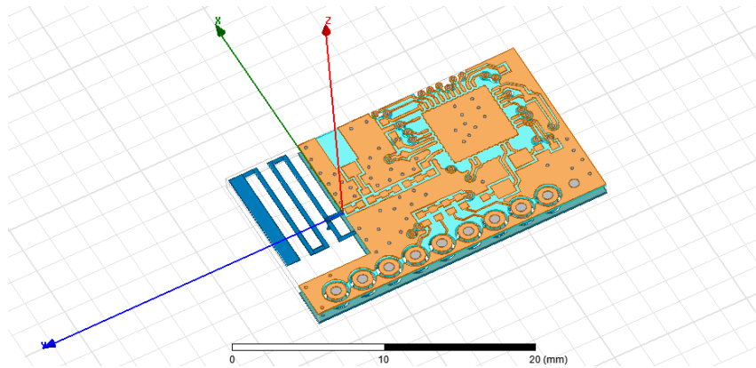
Figure 10. HF-LPT120 天线形式
