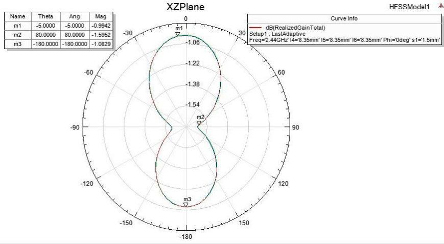
Figure 13. HF-LPT120XZ 平面辐射方向图
