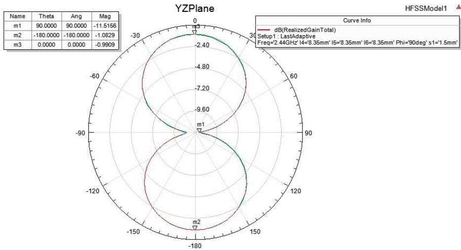
Figure 14. HF-LPT120YZ 平面辐射方向图
