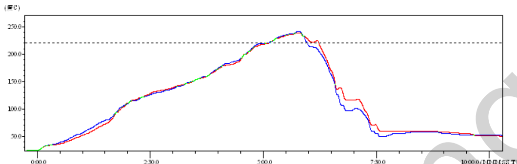
Figure 35. 回流焊焊接温度曲线图
