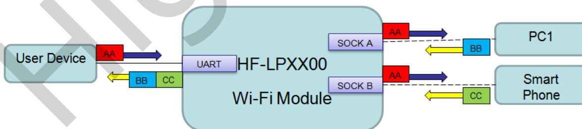
Figure 9. 双 Socket 数据流向示意图
