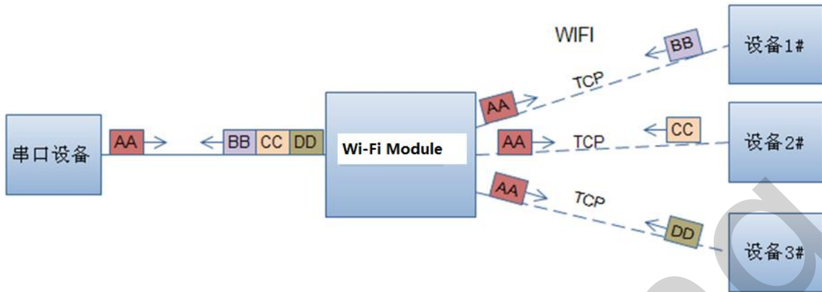
Figure 10. 多 TCP 链接数据传输图示
