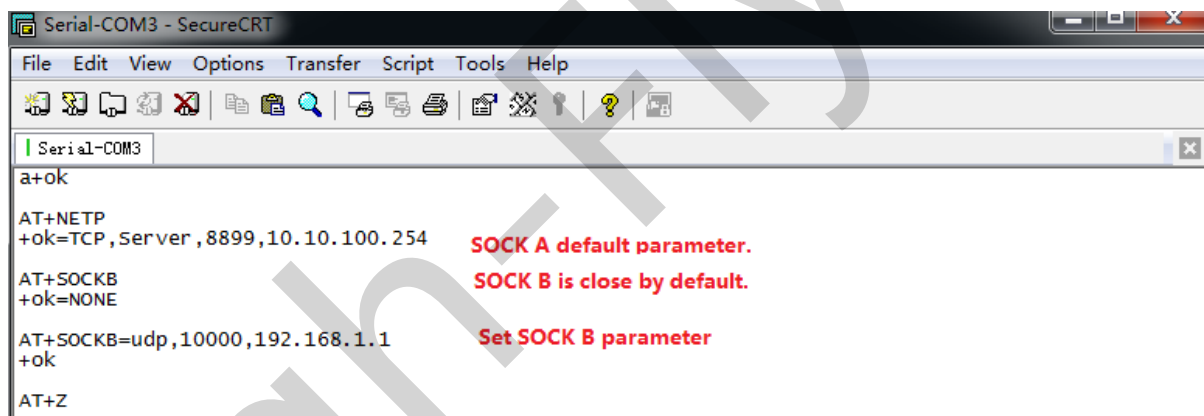
Figure 8. 双 Socket 设置命令
