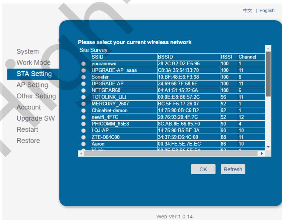
Figure 14. STA Scan Page
