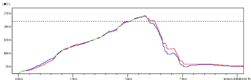
Figure 36. 回流焊焊接温度曲线图
