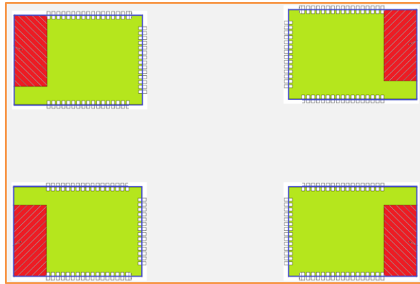
Figure 3. HF-LPB120 模组建议放置区域
