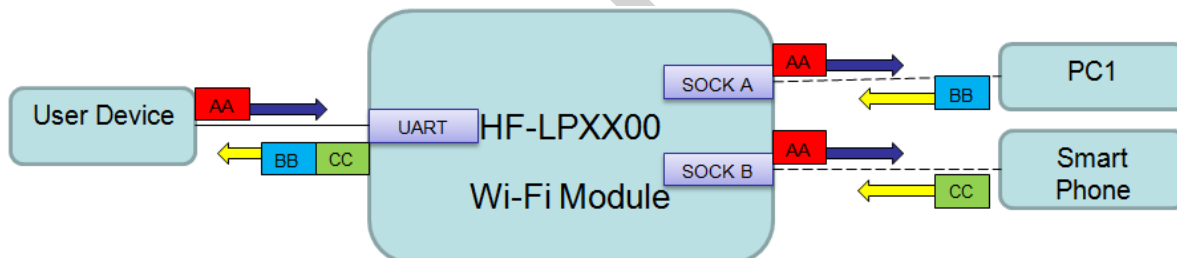
Figure 13. 双 Socket 数据流向示意图
