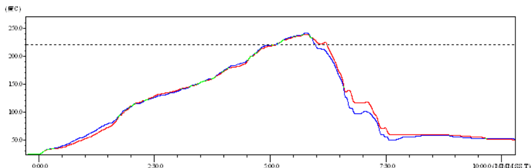
Figure 29. 回流焊焊接温度曲线图
