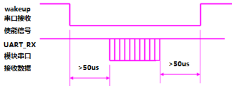
Figure 8. 模块串口接收使能信号示意图
