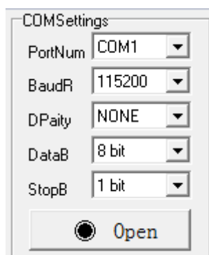
Figure 9. HF-BL300 缺省 UART 参数
