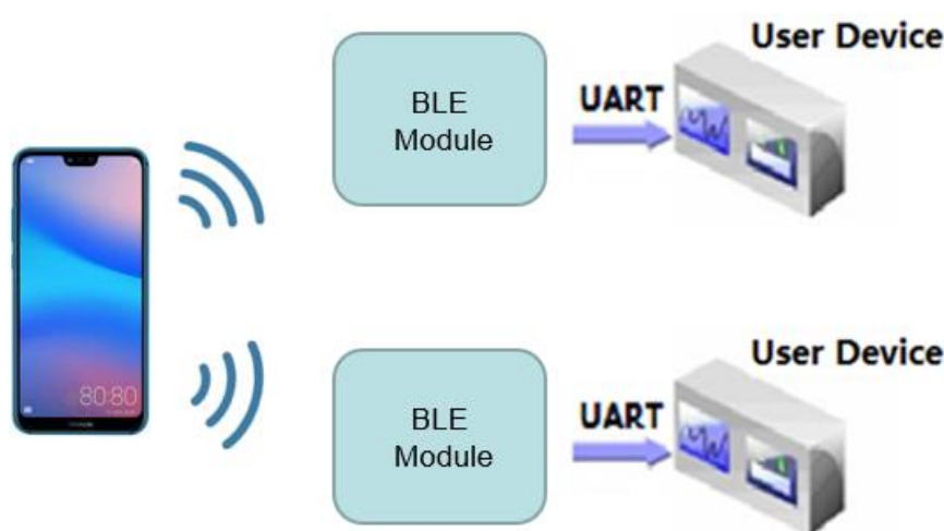
Figure 7. 基本的 HF-BL300 无线组网结构
