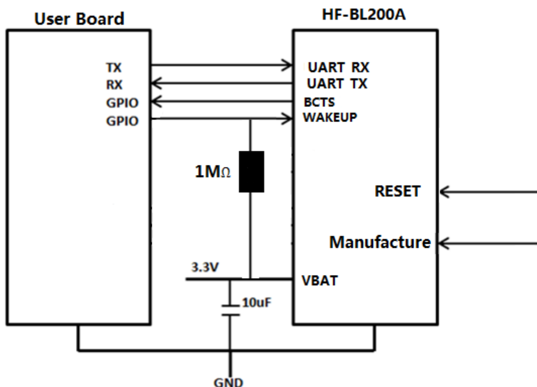
Figure 12. 串口透传典型应用
