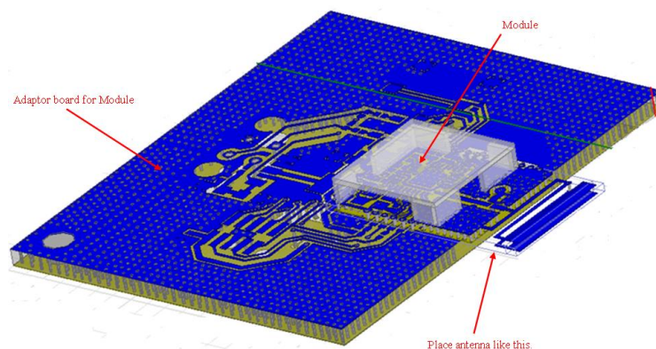
Figure 5. HF-BL300 模块参考放置布局
