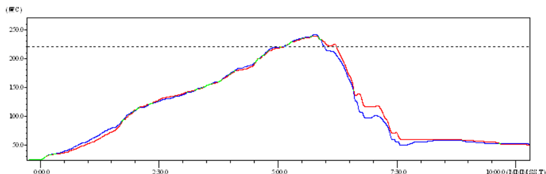
Figure 11. 回流焊焊接温度曲线图
