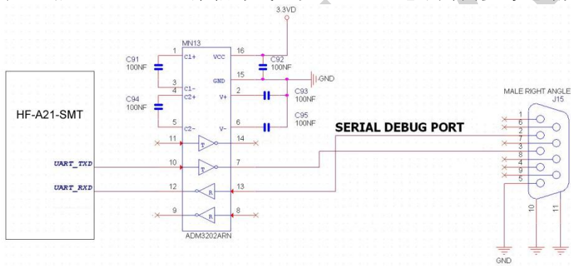
图-11 UART 接口参考设计
