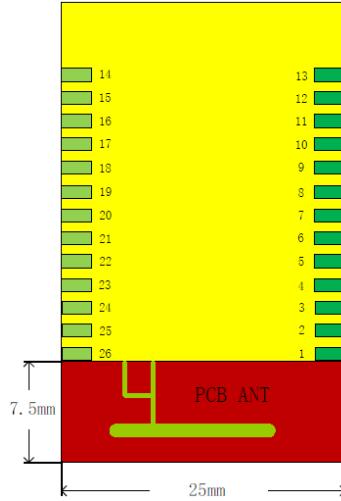
图-4HF-A21-SMT 内置天线禁布区域
