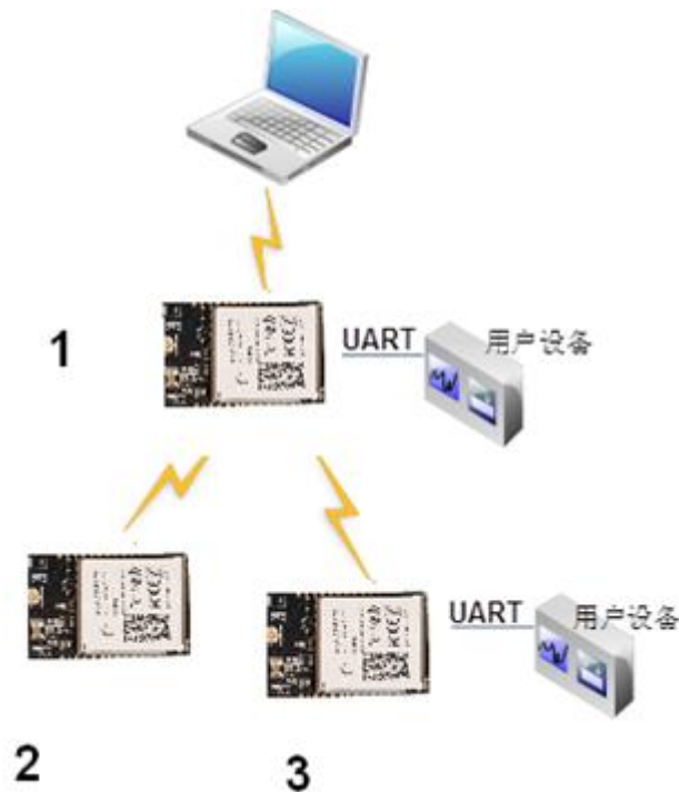
图-16HF-A21-SMT 自组网
