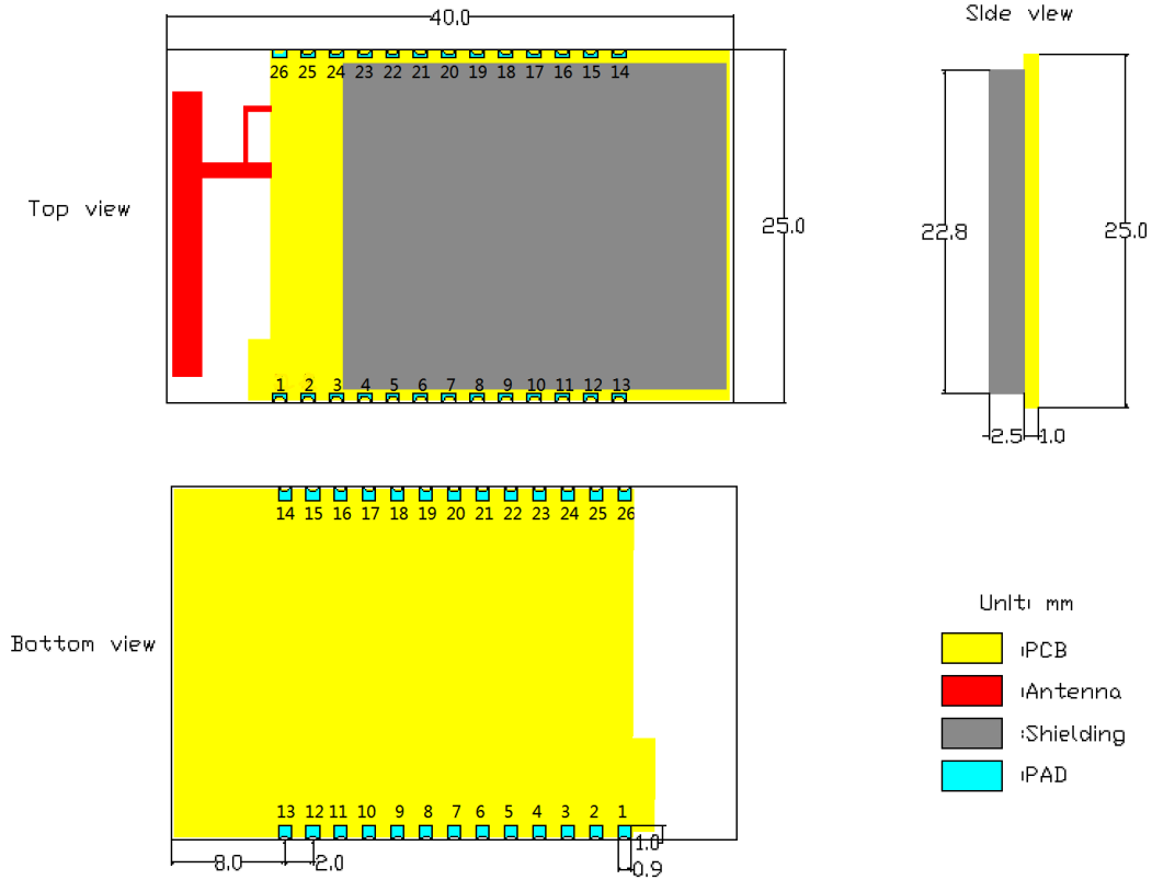
图-3HF-A21-SMT 物理尺寸
