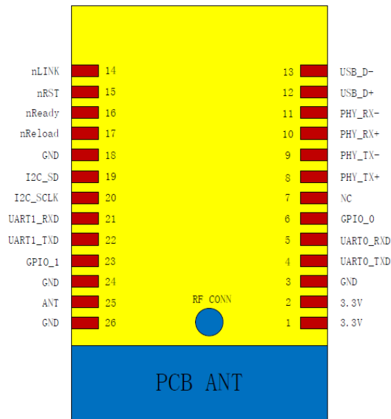
图-2HF-A21-SMT 接口定义
