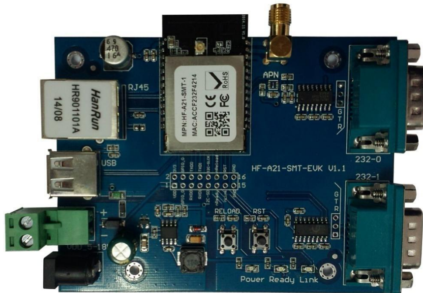
图-6HF-A21-SMT 开发板
