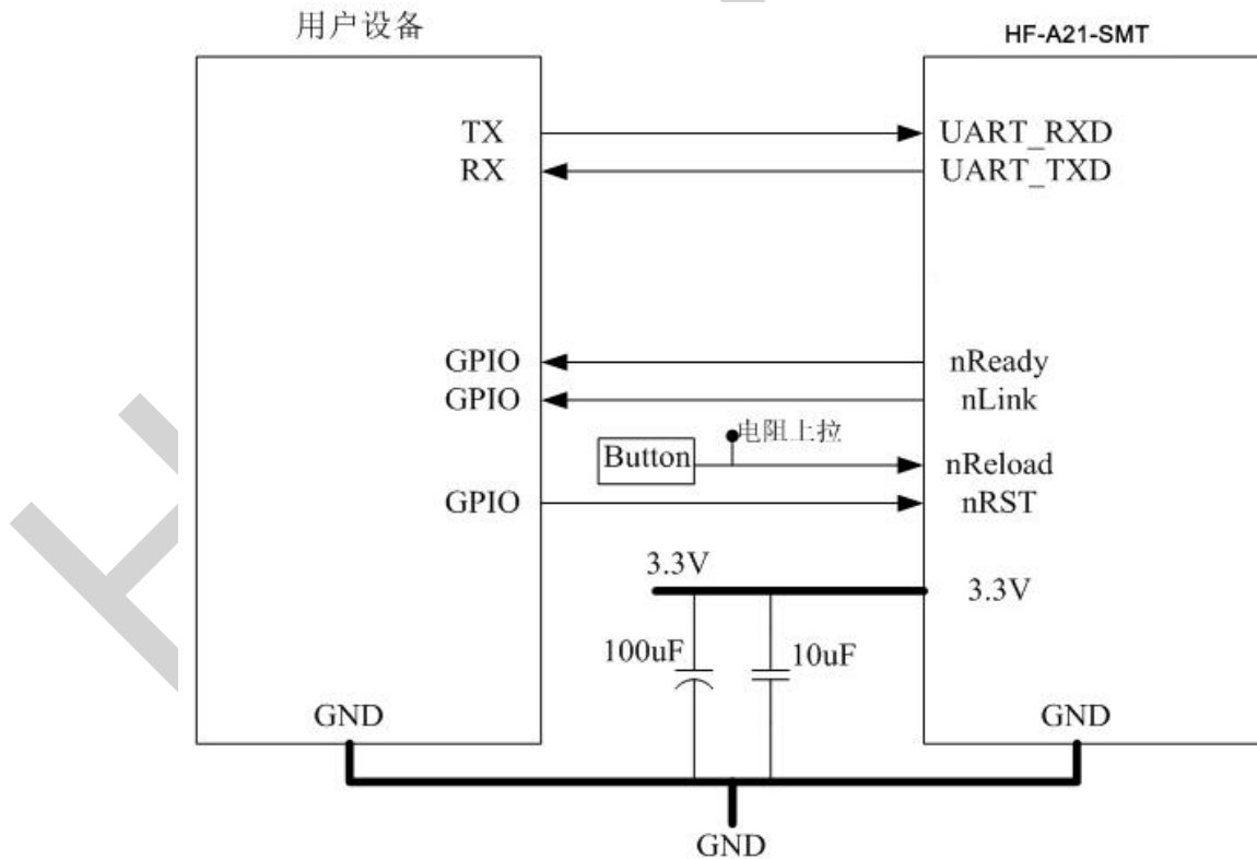
图-8HF-A21-SMT 典型应用硬件连接
