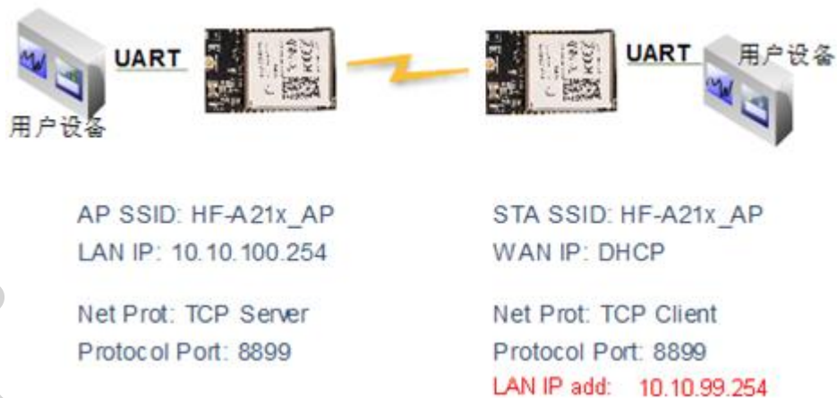
图-39 透明串口应用图示
