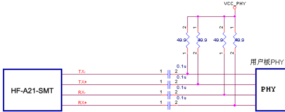
图-10 以太网接口不带变压器方案的参考设计
