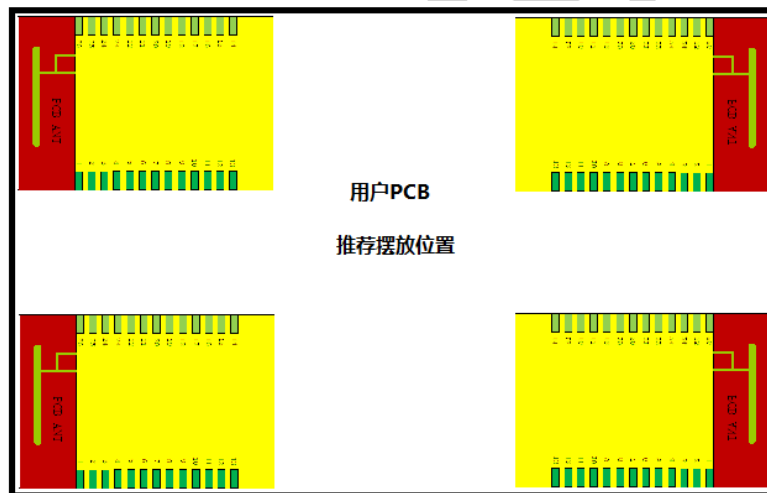
图-5 模组建议放置区域
