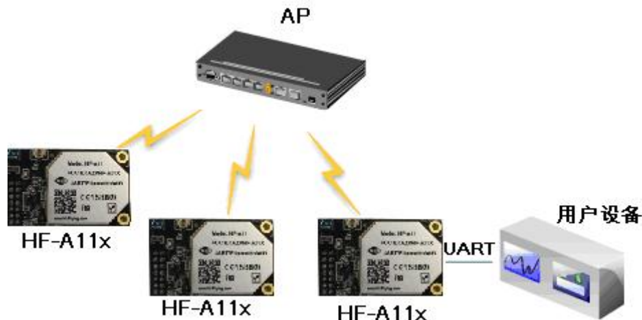
图-15 HF-A11 基础网络组网
