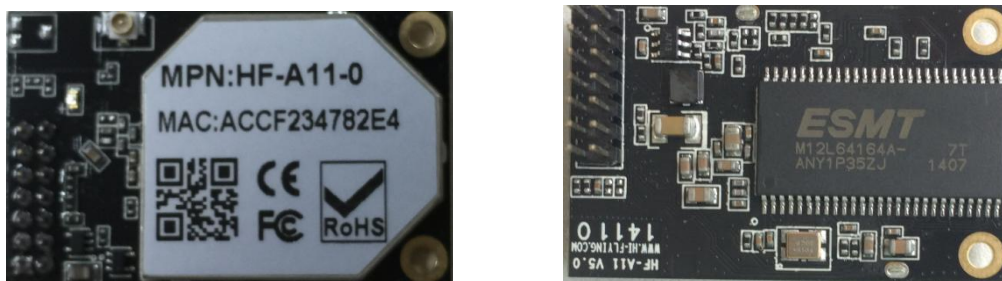
图-1 HF-A11 模块实物图
