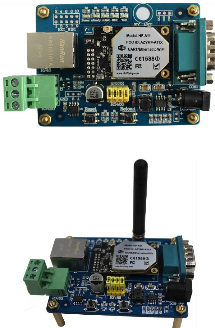
图-6 HF-A11 开发板
