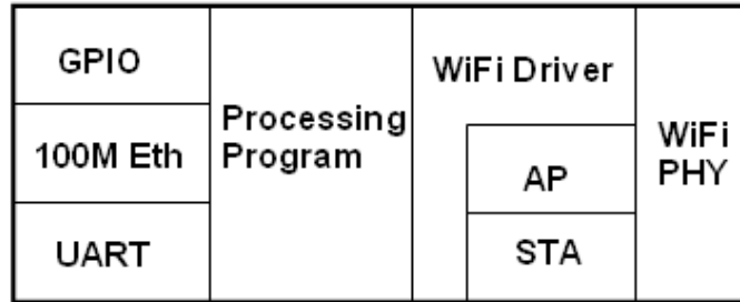
图-14 HF-A11-SMT 功能结构
