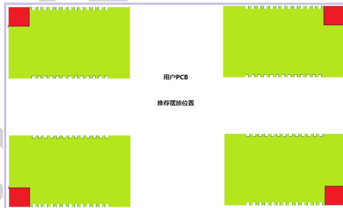
图-5 模组建议放置区域
