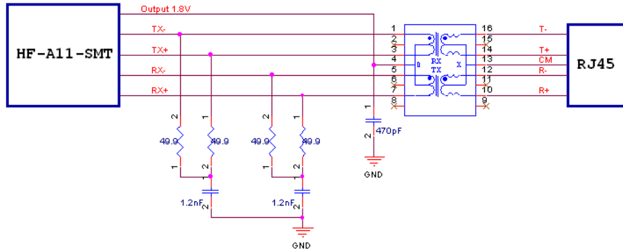
图-9 以太网接口带变压器方案的参考设计
