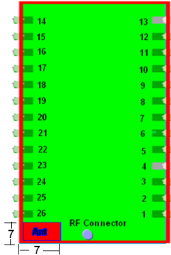
图-4 HF-A11-SMT 内置天线禁布区域
