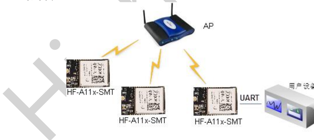
图-15 HF-A11-SMT 基础网络组网
