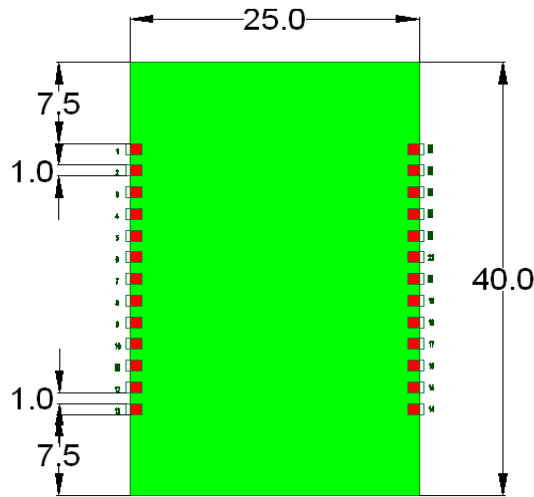
图-3 HF-A11-SMT 物理尺寸
