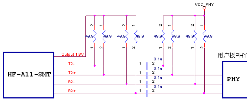
图-10 以太网接口不带变压器方案的参考设计
