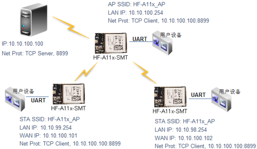
图-40 无线数据采集卡应用图示
