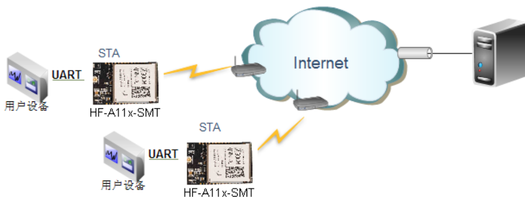
图-38 远程连接应用图示
