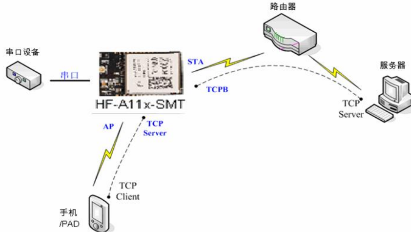
图-17 AP+STA 方式的无线网络
