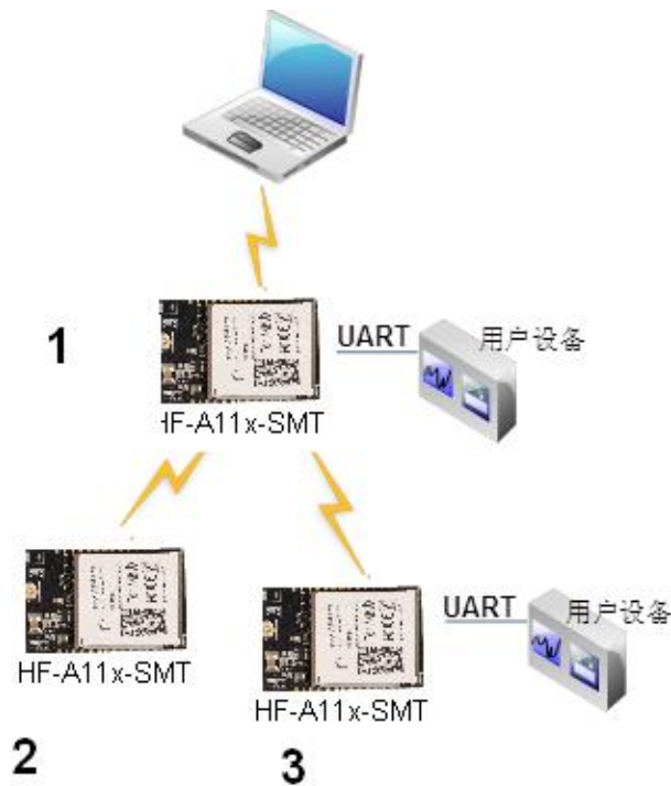
图-16 HF-A11-SMT 自组网
