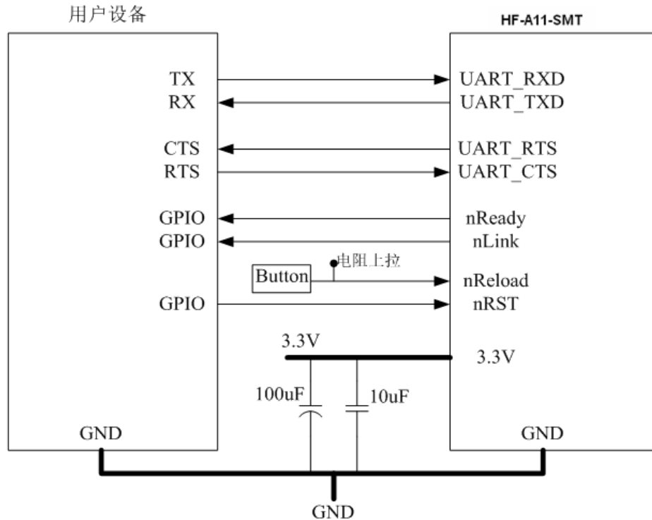
图-8 HF-A11-SMT 典型应用硬件连接
