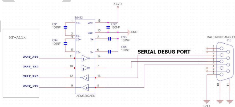
图-11 UART 接口参考设计
