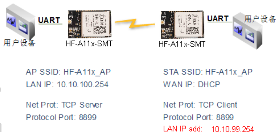
图-39 透明串口应用图示
