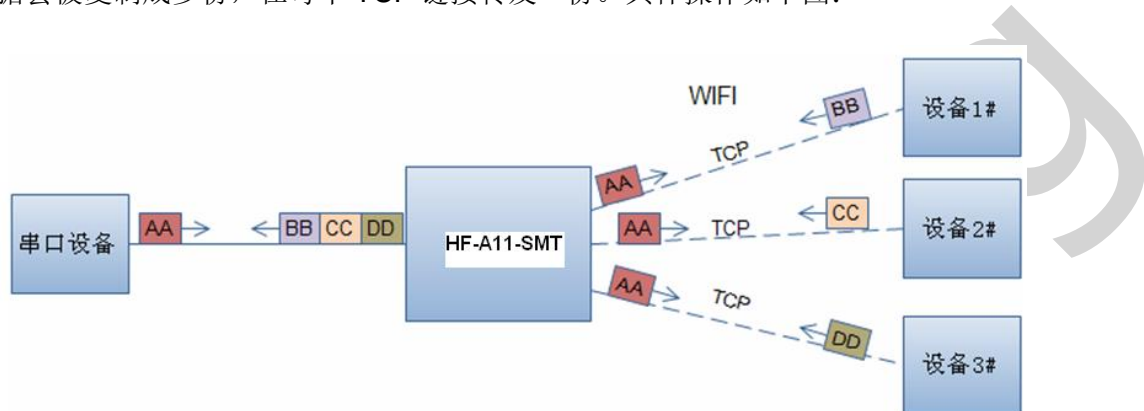
图-13 多 TCP 链接数据传输图示
