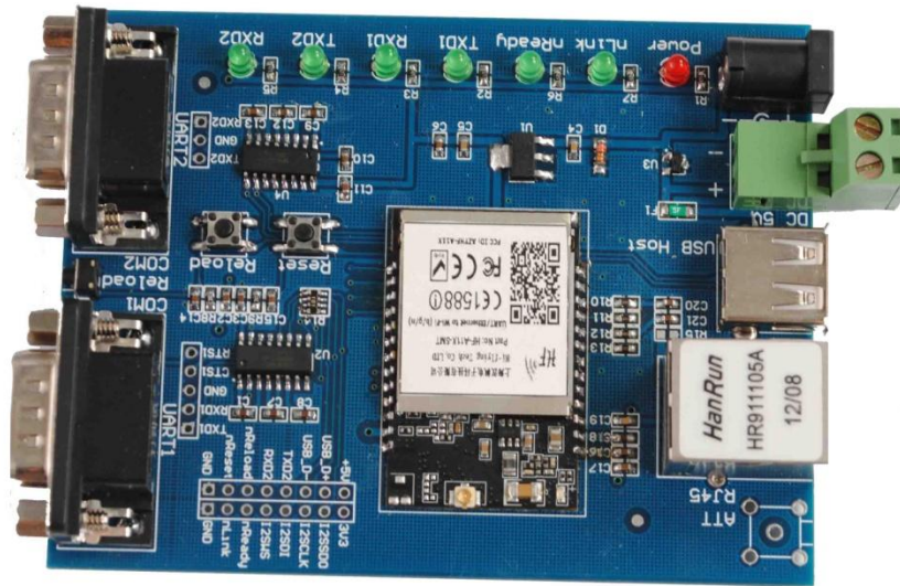
图-6 HF-A11-SMT 开发板
