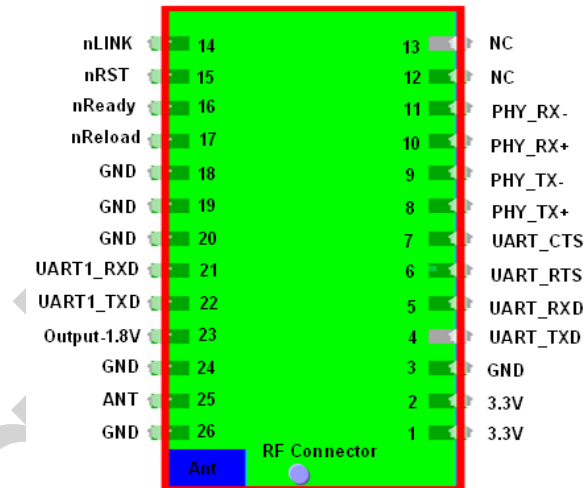
图-2 HF-A11-SMT 接口定义
